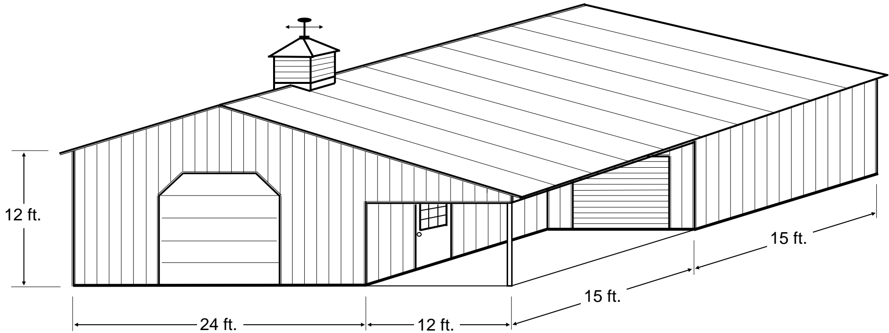
36'x30'x12' w/ 12'x15' Porch
