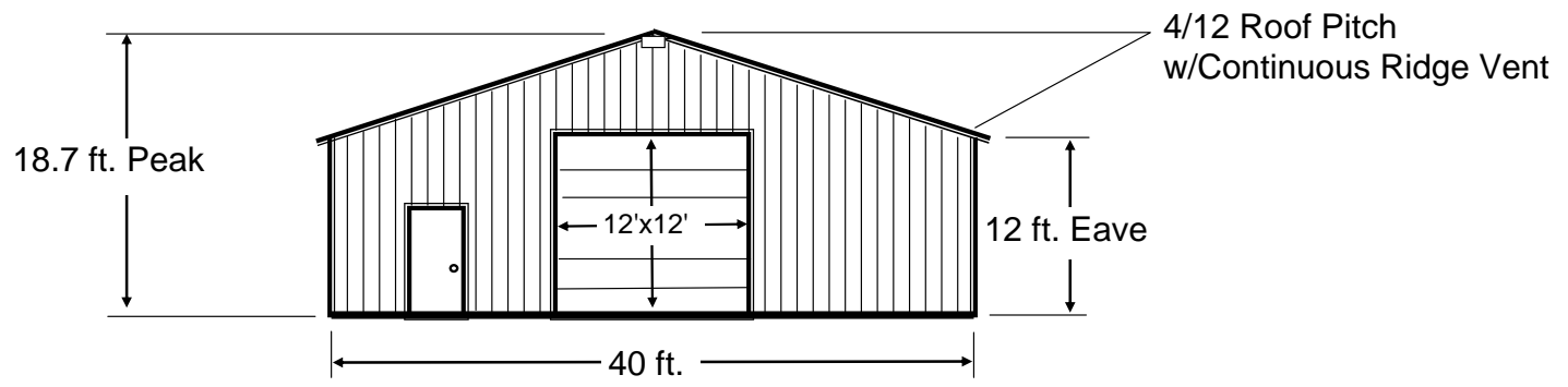
ELEVATION
